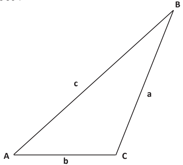
Obtuse Oblique Triangle
